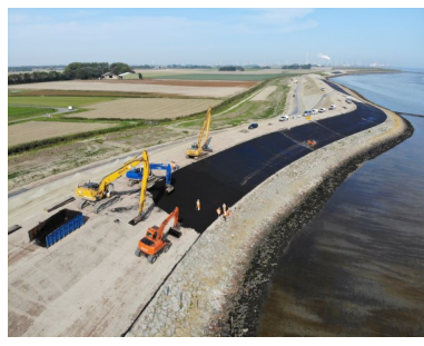
Op grote delen van de dijk komt asfalt op de buitenzijde.
